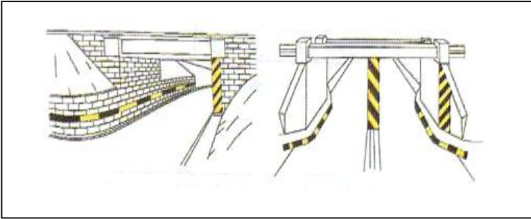
marcaje pe ziduri de sprijin și pe infrastructurile pasajelor inferioare
